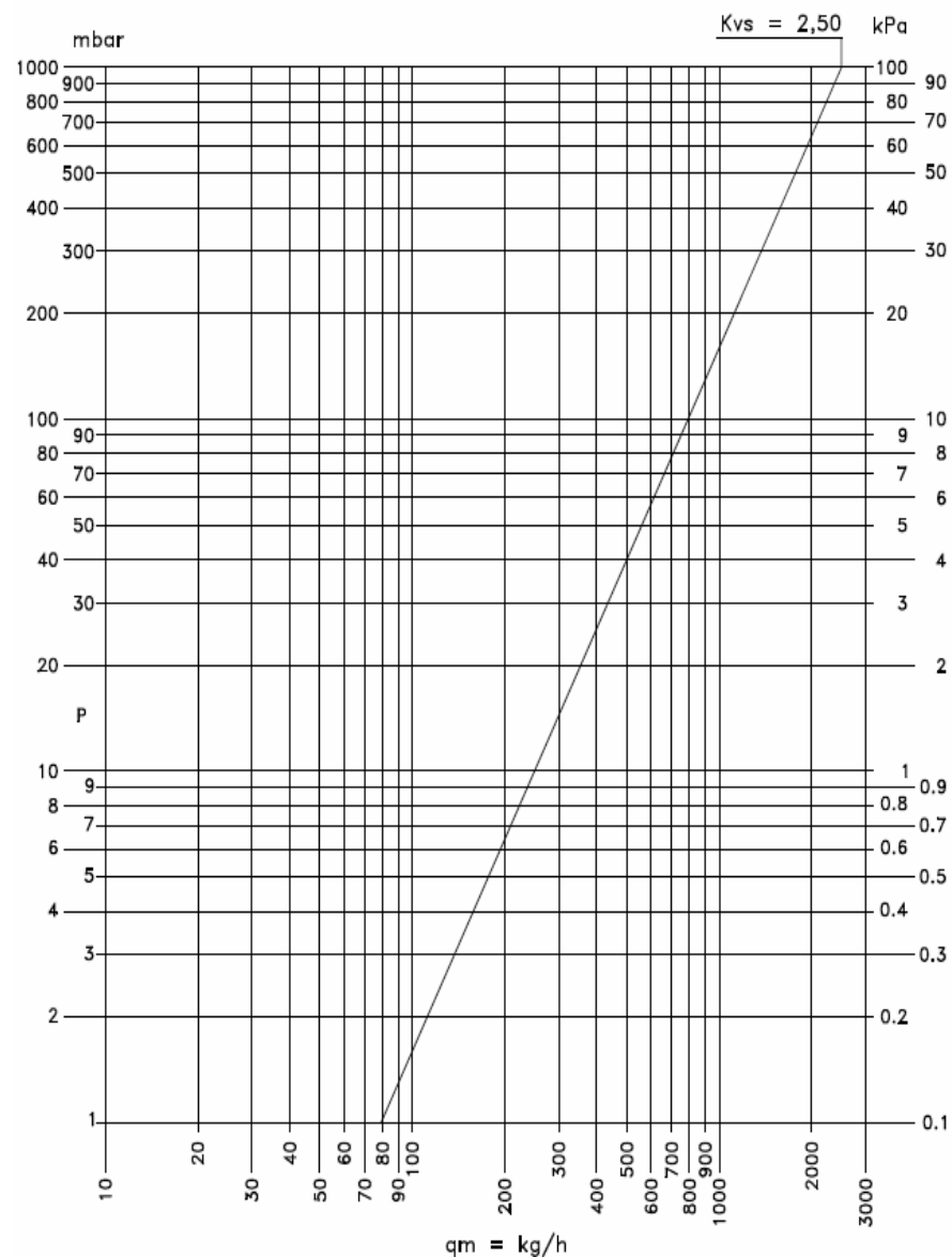
9. График пропускной способности регулировочного клапана
